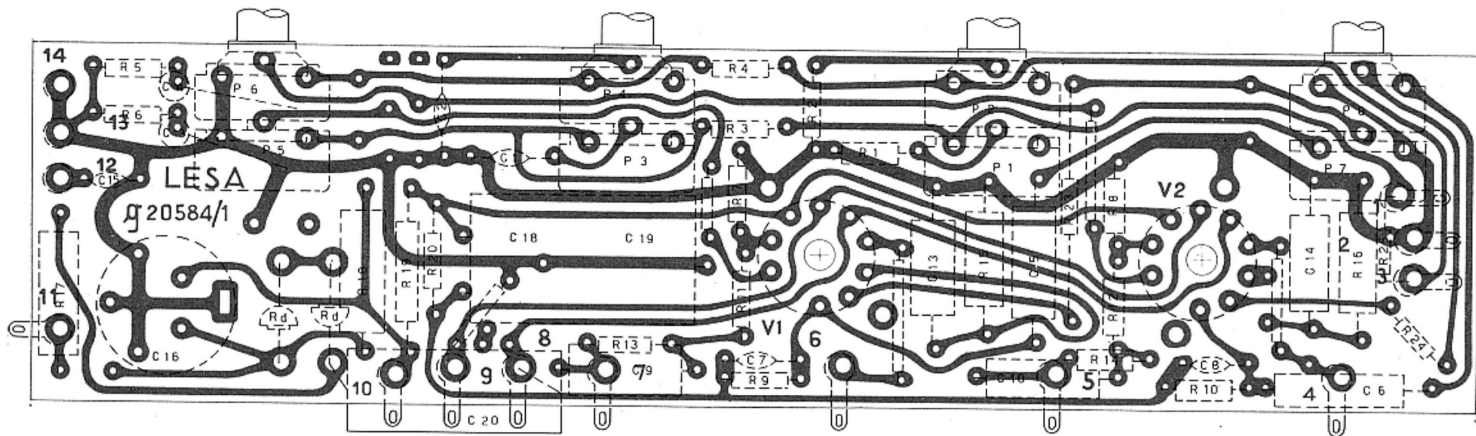
Circuito stampato
